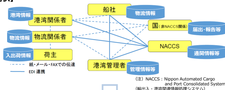
図表1 《港湾システム最適化のイメージ図》
