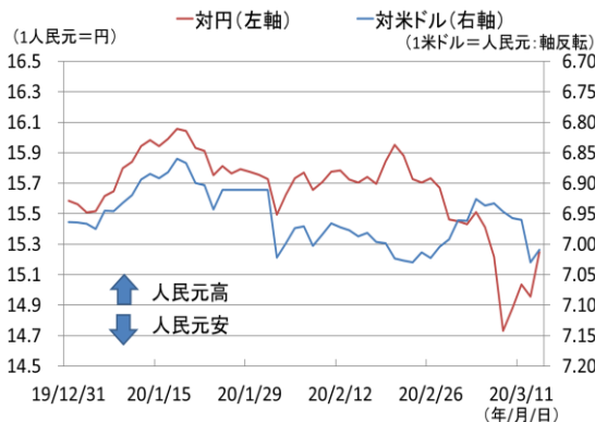
【図表3】人民元の対円、対米ドルでの推移(2019/12/31~2020/3/13)
